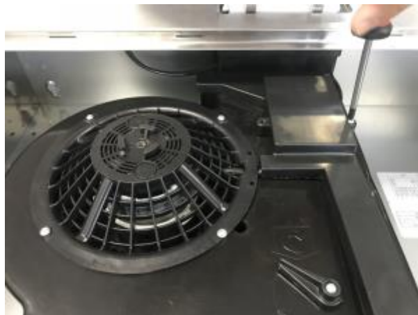
1 - Kreuzschlitzschrauben lösen
